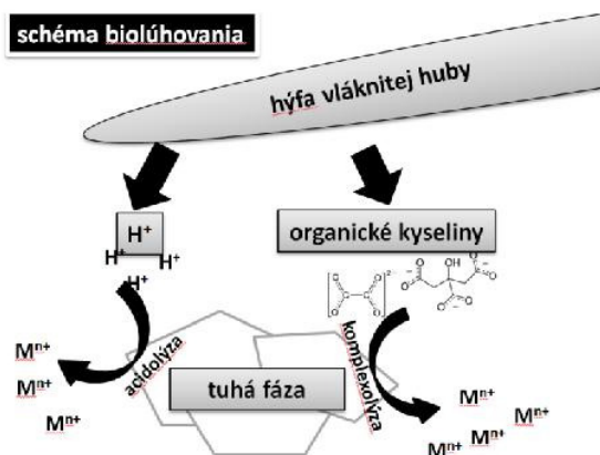
Obr. 1 Schéma uvoľňovania kationov kovov z povrchov pôdnych častíc a minerálov účinkom kyslých vodíkov a organických kyselín produkovaných mikroskopickou vlákňitou hubou.
