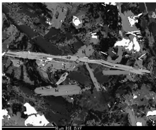
Obr. 4 Mikrofotografia lamprofyru, čísla analyzovaných amfibolov odpovedajú číslam v tab. 2, (odrazené elektróny), elektrónový mikroanalýzátor, lokalita: Martinské hole
