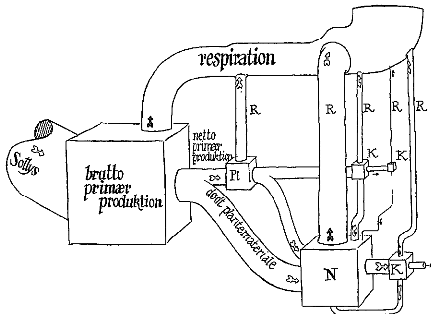
Fig. 45. En lidt mindre skematisk fremstilling af energistrømmen gennem et naturligt økosystem. Her svarer kassernes størrelse til størrelsen af biomassen på de enkelte trofiske niveauer. Rørenes tykkelse svarer i grove træk til størrelsen af den energistrøm, der foregår mellem de dele af systemet som rørene forbinder.
