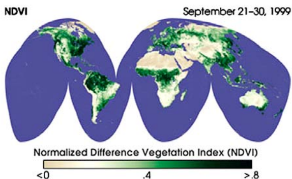
Figur 4 NDVI fra hele Jorden. Kilde: Earthobservatory, NASA.
