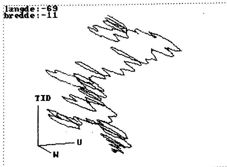
Fig. 13. Pendul med gnidning og hvid støj.
