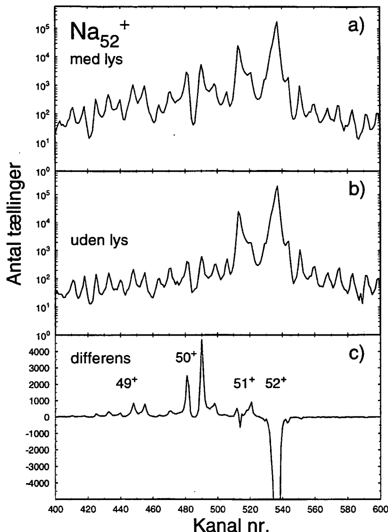
Figur 5.1: \text{Na}_{52}^{+} -massespektrum. Kanalnumrene på x-aksen afspejler den position på tælleren hvor klyngen har ramt. Opløsningen er givet ved de enkelte toppe, der hver svarer til en strip på printpladen (jfr. appendiks D). Der går således ca. 8 kanaler på en strip.
