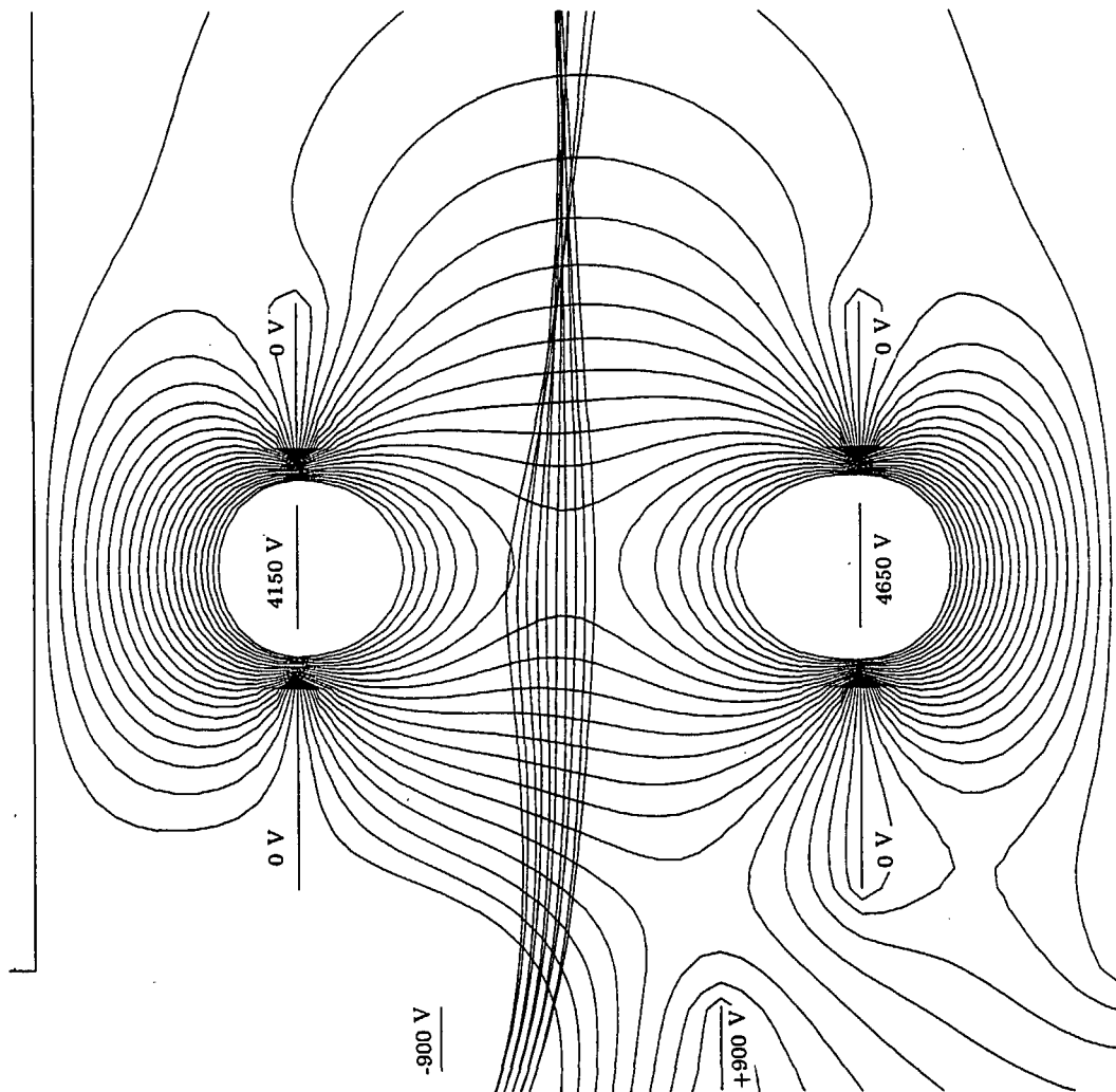
Figur C.8: \text{Na}^+_{45} med fire døtre i Einzel-linsen. Beamene kommer ud af energi-filteret i bunden af billedet. De to baner yderst til højre definerer moderbeamet. Endvidere er indtegnet ækvipentialkurver for hver 100 volt fra 100-2000 V.
