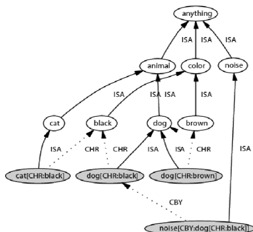
Fig. 1: Ontologi/taksonomi over simple begreber (hvid baggrund) med fire sammensatte begreber, fra den udvidede generative ontologi, indsat (grå baggrund).
