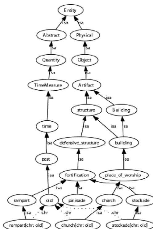
Fig. 2: Udsnit fra en WordNet-baseret ontologi
