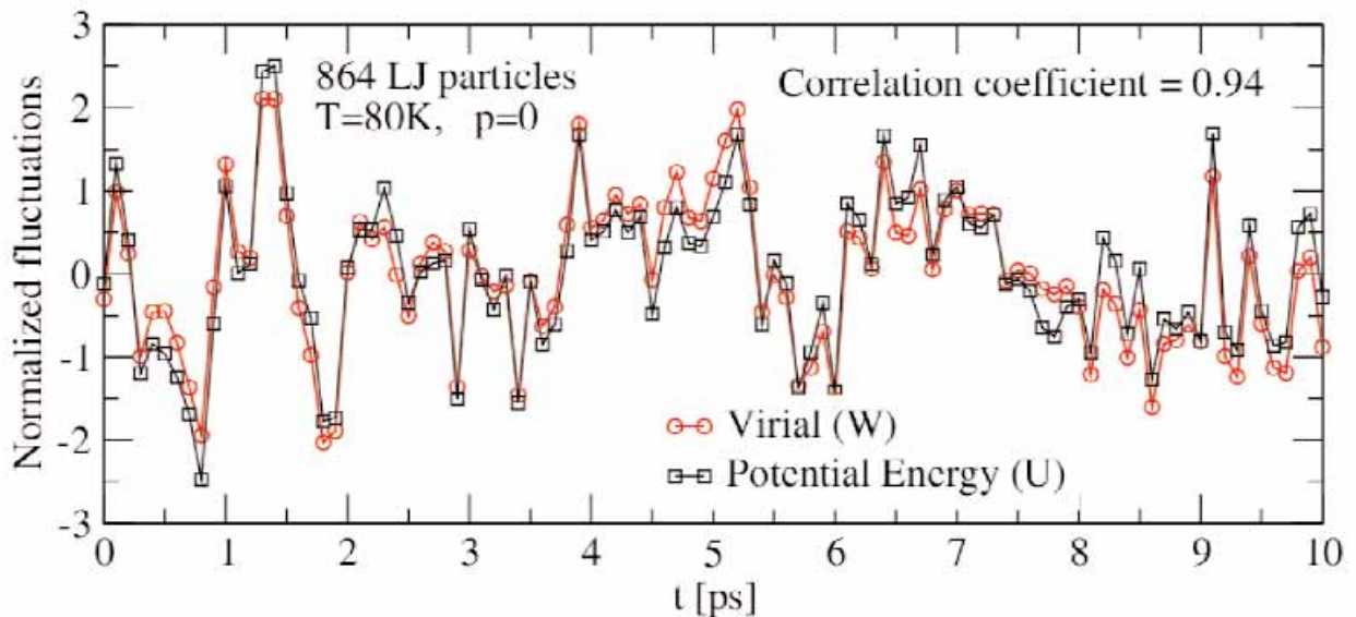
Figur 1: Tryk og energifluktuationerne af Lennard-Jones væsken som funktion af tiden. Mere præcist er det der er plottet de såkaldte konfigurationelle bidrag (henholdsvis "Virial" og "Potential Energy"). Figuren er taget fra [1].
