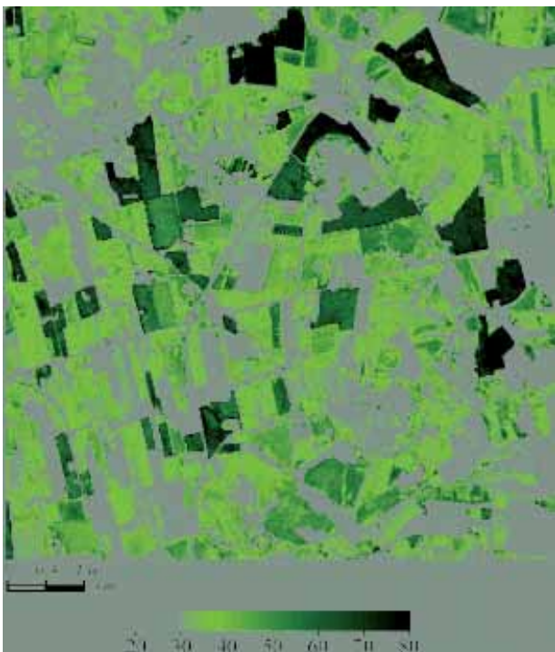
Figur 1. For at kortlægge kvælstofindhold blev der anvendt jordobservationer fra satellitten SPOT, der har en rumlig opløsning på 10 m.
