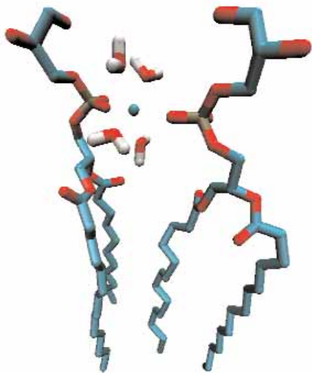
Figur.2. Computersimulering af hvordan calcium (i cirklen) organiserer sig ved binding til lipider (lange rød/turkise molekyler) og vand (små rød/hvide molekyler). Strukturen er klippet ud af en simulering med mange molekyler (se fig. 1) og viser den grundlæggende påvirkning af dette metal på membraner. Det er foreslået at dannelsen af denne struktur er grundlaget for flere af calciums biokemiske funktioner.
