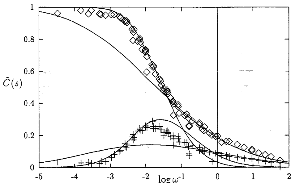
Figur 3.5: Modelfunktionen (de fuldt optrukne kurver), fittet individuelt til henholdsvis hørfrekvens- ( \log(\omega) > 0 ) og lavfrekvens-området ( \log(\omega) < -2 ). Parameterværdierne er som angivet i teksten.
