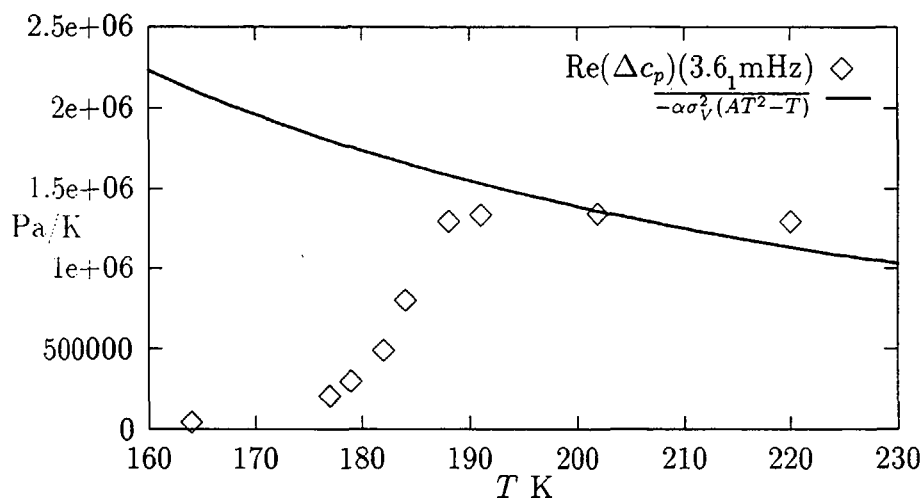
Figur 6.2: Den konfigurationelle del af varmekapaciteten. Fit til eksperimentelle data aflæst fra [Chr 89 s. 139]. A = 0.05 1/K og \alpha\sigma_V^2 = -4.0 \pm 0.4 \times 10^{-10} Pa -1 . Bemærk at der er tale om den volumen-specifikke varmekapacitet.
