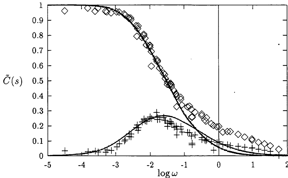
Figur 3.3: Fitning af modellen til masterkurven med T = 186,8\text{K} ; de benyttede parameterværdier er: \sigma_E^2 = 7.56 \times 10^4\text{K}^2 , \mu_E = -2.02 \times 10^4\text{K} og \tau_0 = 2.2 \times 10^{-47}\text{s} .
